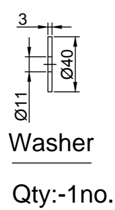
Washer Qty:-1no.
