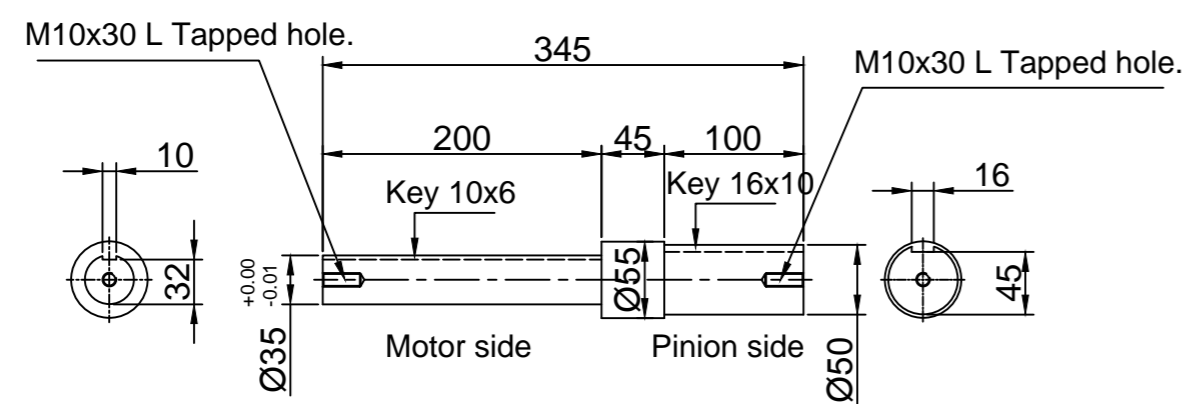
SHAFT Qty:-1no.
