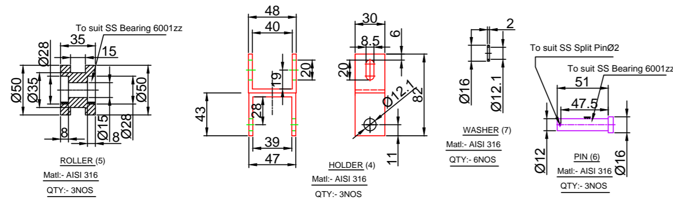
ELEVATION
