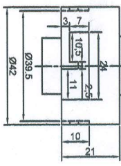
② SPINDLE ASIS 316L (IS 1570-07C19N6M02T28) Qty:- 1No.
