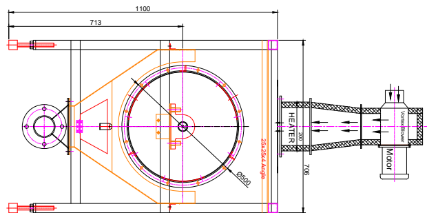
L. SIDE VIEW
