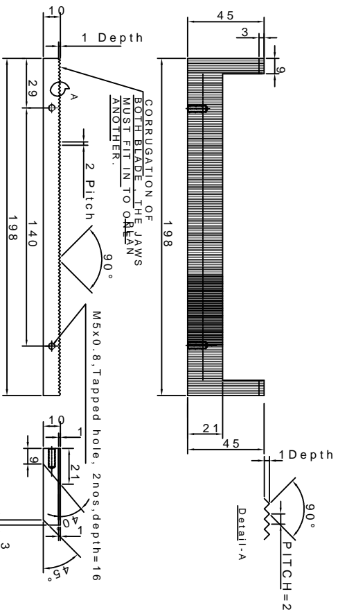
ELEVATION
