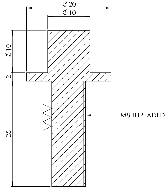
SECTION A-A SCALE 3 : 1
