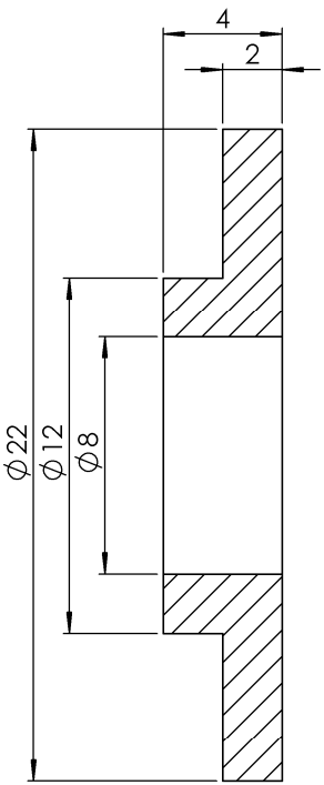
SECTION A-A
